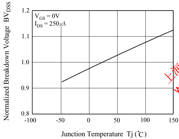
Fig3. BV_{DSS} - T_j
