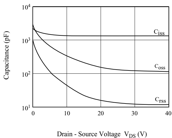
Fig 7. C - V_{DS}
