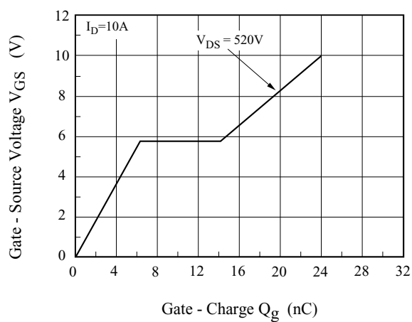
Fig8. Q_g - V_{GS}
