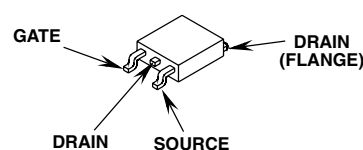
JEDEC TO-252AA
