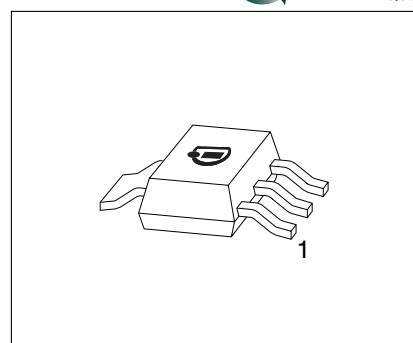
PG-SOT-223
