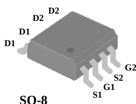
SO-8
