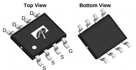
SOIC-8
