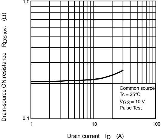
R_{DS(ON)} - I_D
