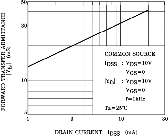
|Y_{fs}| - I_{DSS}
