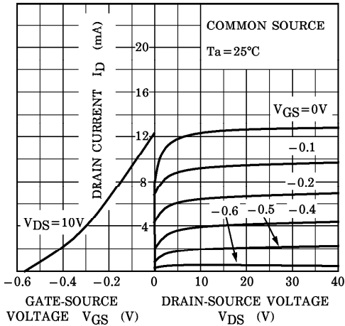
I_D - V_{GS}
