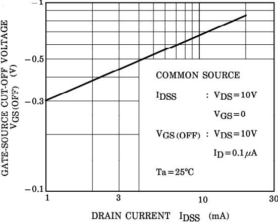
V_{GS(\text{OFF})} - I_{DSS}
