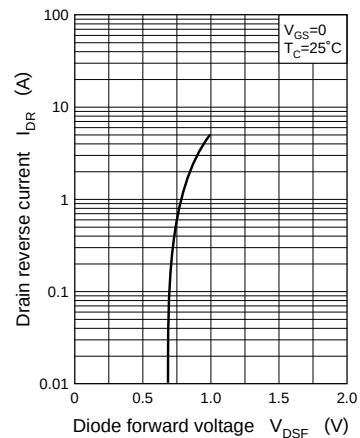
I_{DR} - V_{DSF}
