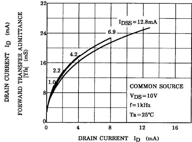
|Y_{fs}| - I_D
