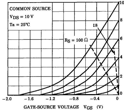
I_D - V_{GS}
