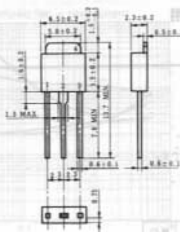
2SJ133外形図
