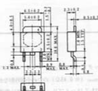
2SJ133-Z外形図
